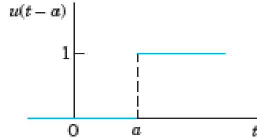
Fig. 119. Unit step function u(t-a)
