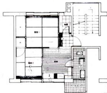
51C型平面図／吉武泰水＋郭茂林 (1950) 床面積39.00㎡
