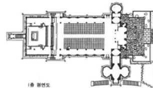
1층 평면도
