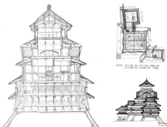
마츠모토성(松本城) 천수각(복합연립식)
