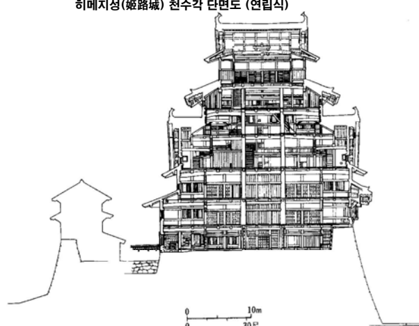
히메지성(姫路城) 천수각 단면도 (연립식)
