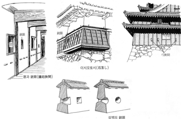
성의 방어시설
