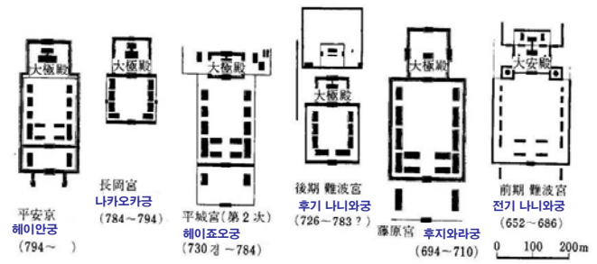
고대궁실 배치복원도
