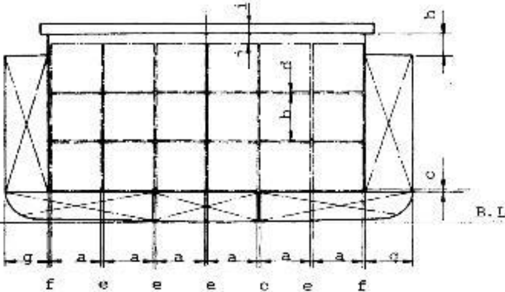
400TEU 급 세미 컨테이너선의 화물창 단면도
