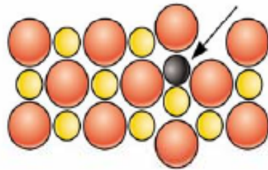
Frenkel 결함
