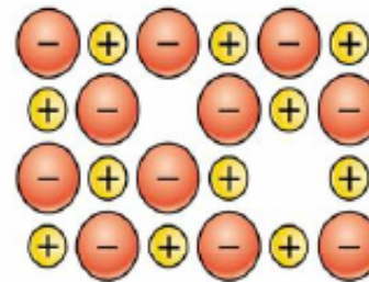
Schottky 결함
