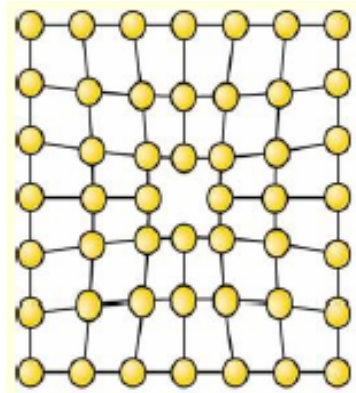
Vacancy 결함
