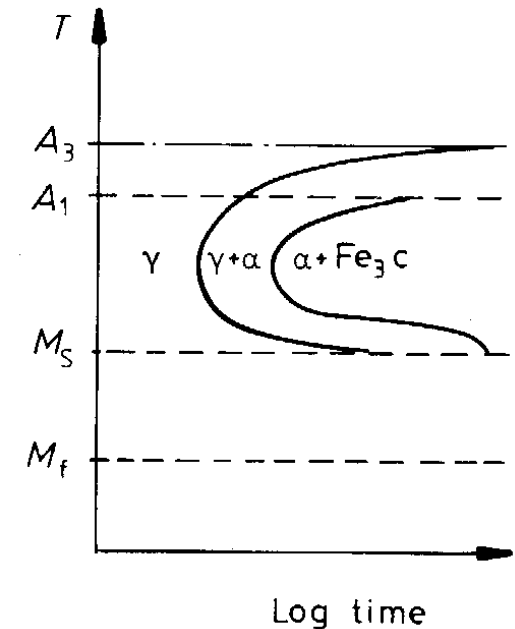
(d) C_0 합금의 TTT curve
