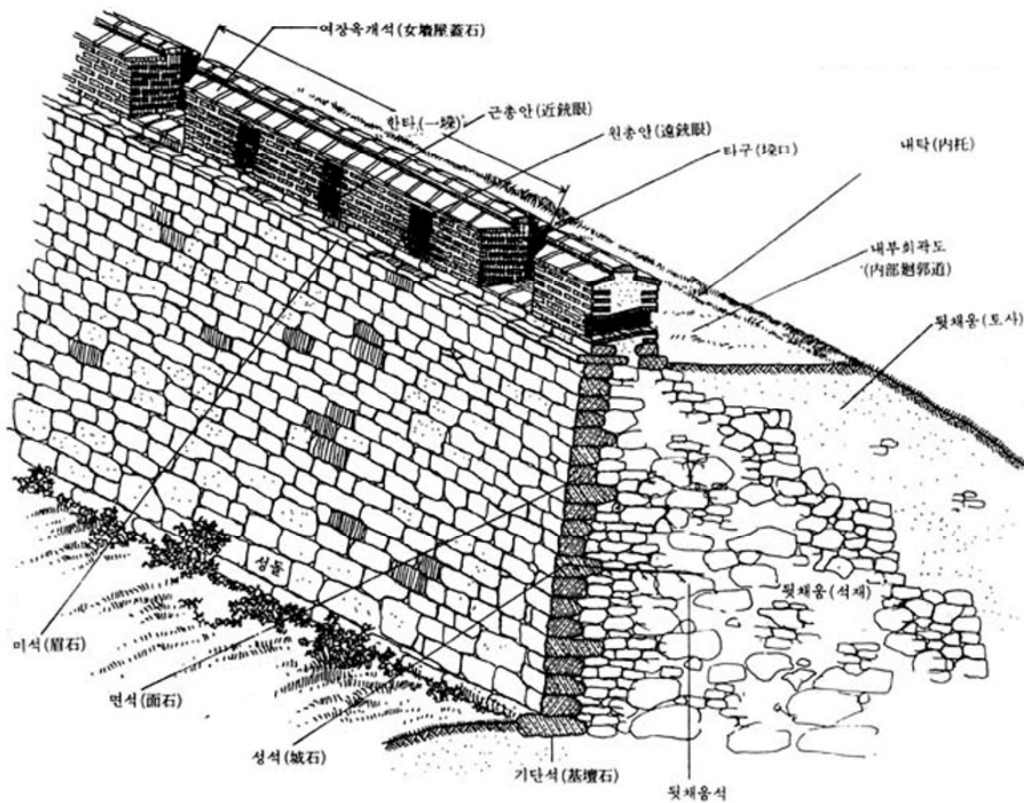
성벽의 구조
