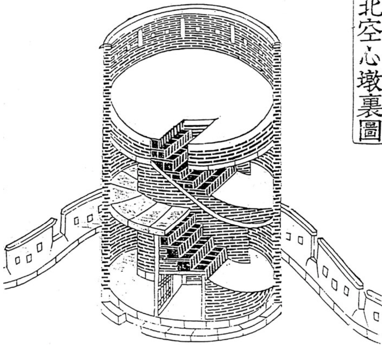
東北空心墩裏圖 〈華城城役儀軌〉
