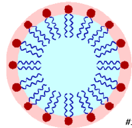
a micelle
