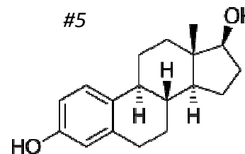
E2
