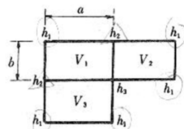
사각각주법
