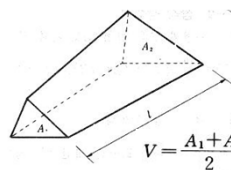
양단면적 평균법 V: Soil Mass (m³) 실제 토량보다 크다
