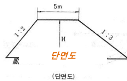
(단면도)
